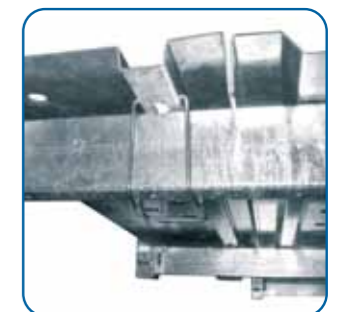
Chapas de extensible con clip de montaje rápido Extension floor plates with quick mounting clips
